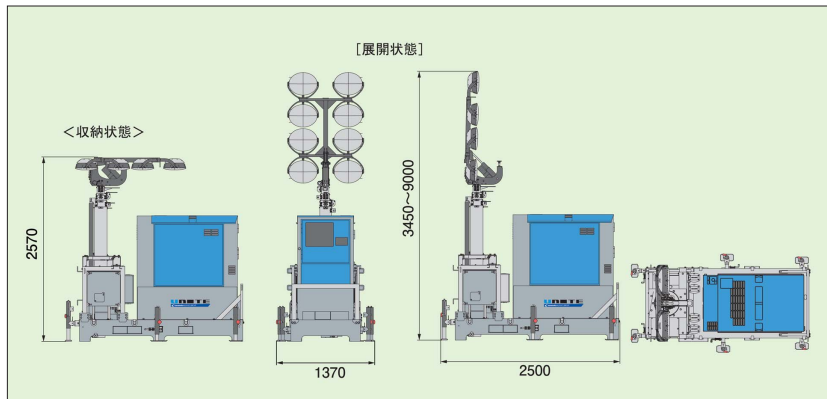
■外形寸法図(単位:mm)
